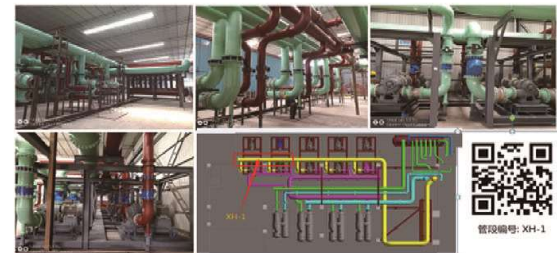
工厂化预制加工和二维码编码图一
