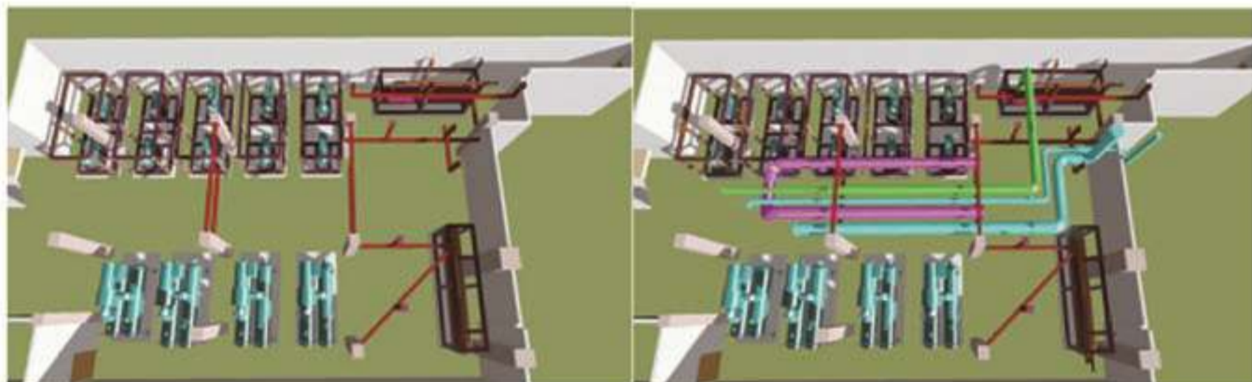
机房模块及管道装配---BIM模拟装配图二 上层主管安装
