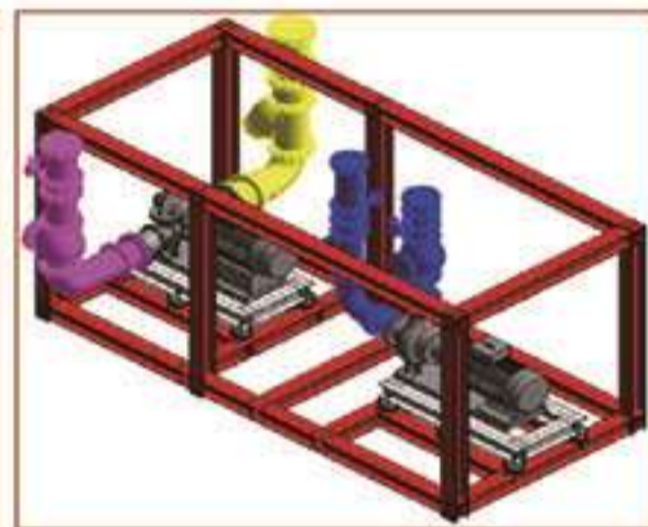
BIM机房管线及设备分段与集成预制加工模型图六
